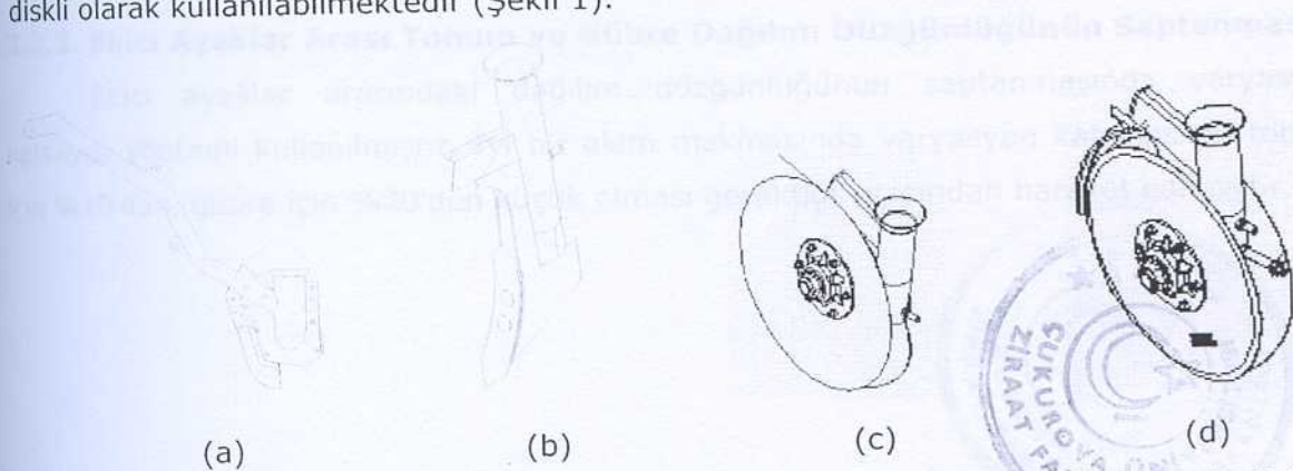
Şekil 1. Ekim makinasında kullanılan çizi açıcı ayak tipleri (a-balta, b-çizel, c-tek disk, d-çift disk)
